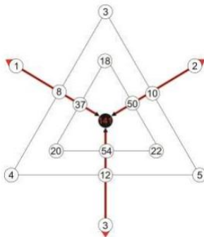
Asteroide 141
