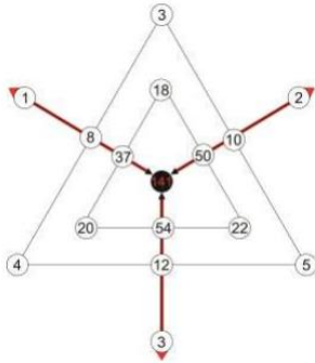
Asteroide 141
